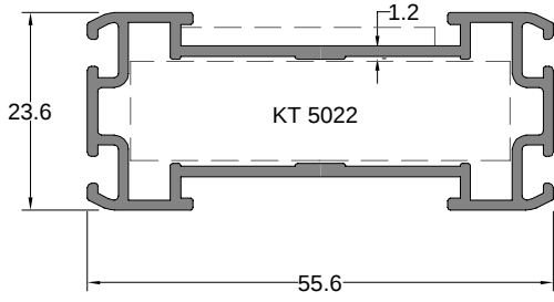
Düşey Yatay Profil MULLION PROFILE
