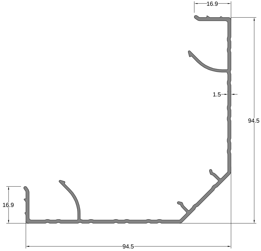
90° Köşeli Dönüş Profili 90° CORNER RETURN PROFILE
