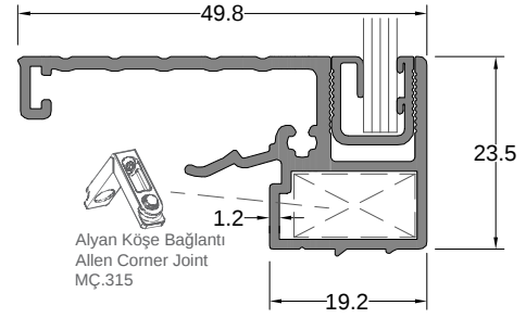
Tırnaklı Kaset Profil CASSETTE PROFILE
