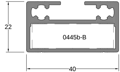
Kapı Kanat Profil DOOR SASH PROFILE
