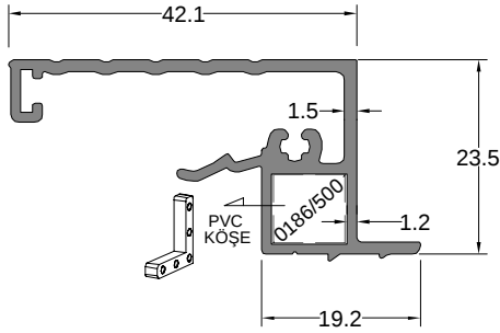
Yapıştırma Kaset Profil GLUING CASSETTE PROFILE
