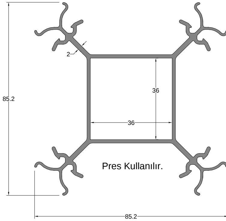
Köşe Birleşim Profili CORNER JOINTING PROFILE
