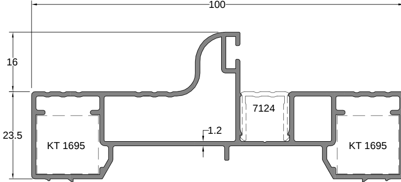
Kapı Kasa Profil DOOR FRAME PROFILE
