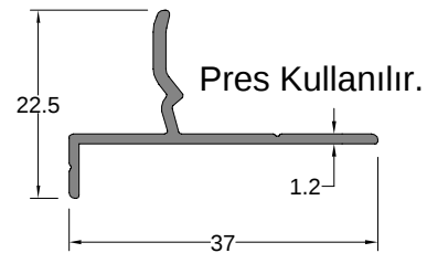
Ahşap Panel Bağlantı Profil WOOD PANEL CONNECTION PROFILE
